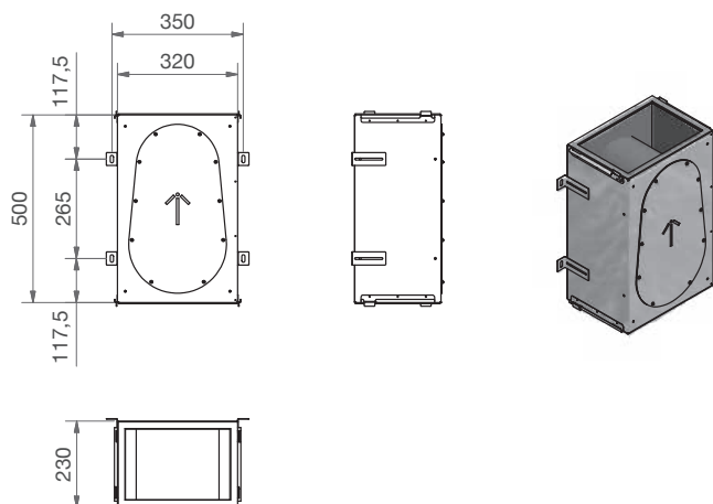
CW-P 320 Plaque d'extrémité DN125
