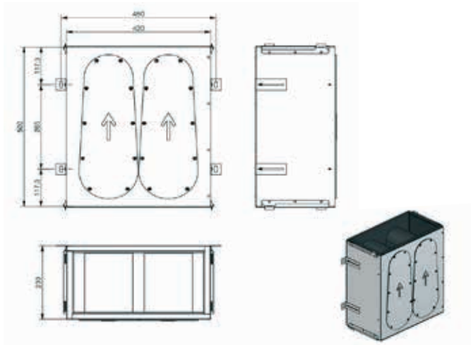
CW-P 420 Plaque d'extrémité DN160
