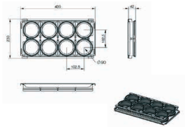
CW-P 320 Plaque d'extrémité DN180
