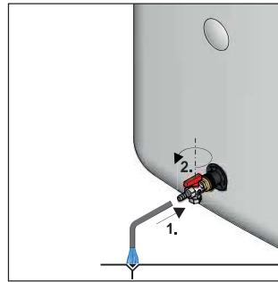
Fig. 5-1 Processus de vidange sans p=0 système solaire
