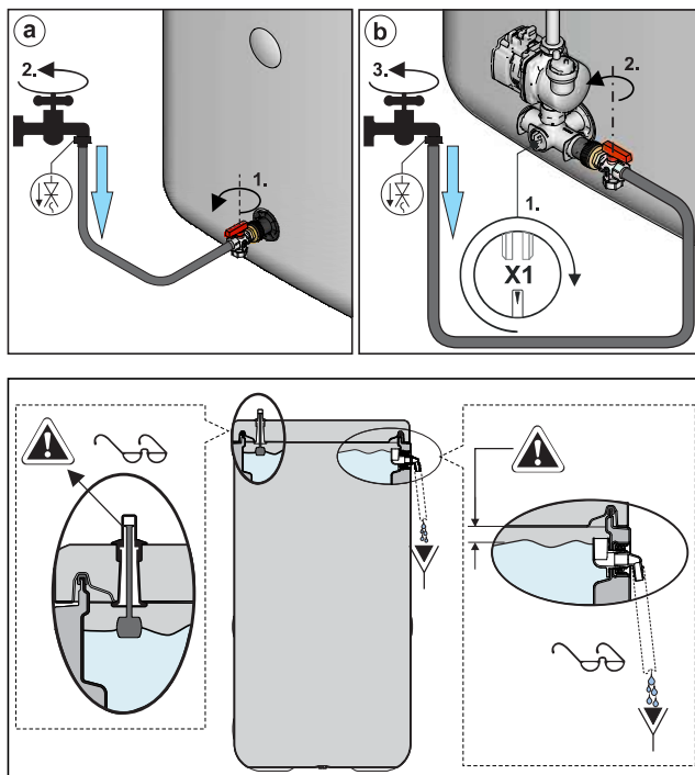
Fig. 3-3 Montage du flexible du tuyau d'évacuation sur le trop-plein de sécurité
