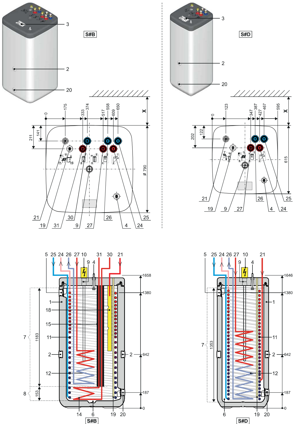
Fig. 2-1 Raccordements et dimensions, Ballon d'eau chaude haute performance avec appoint solaire - p=0 Type EKHWP 300/500B
