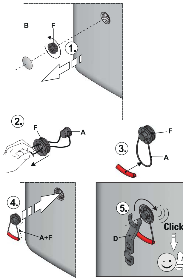
Fig. 3-1 Montage des poignées
