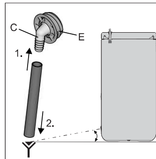
Fig. 5-3 Étape 1
