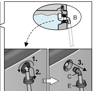
En option : démonter la pièce de raccordement du trop-plein de sécurité
