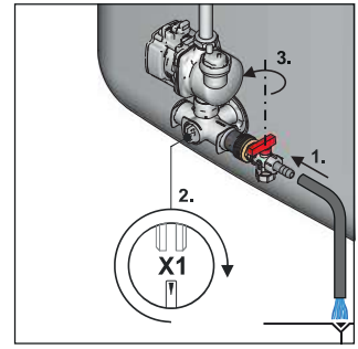
Fig. 5-2 Processus de vidange avec p=0 système solaire
