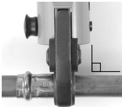
Figure 7 – Mâchoires tenues à l'équerre du raccord
