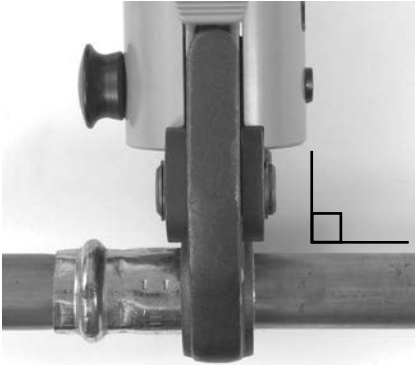
Abbildung 7 – Backen gerade am Fitting
