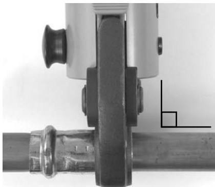
Obrázok 7 – Čeluste usporiadané kolmo na tvarovku
