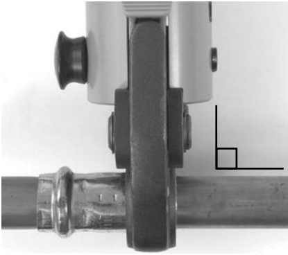
Figura 7 – Colocar os mordentes alinhados no engaste
