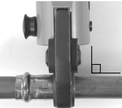
Figuur 7 – Bekken loodrecht op de fitting
