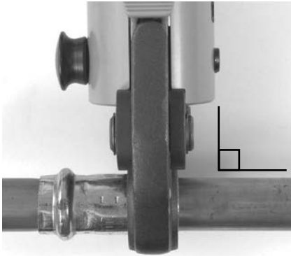
Figura 7 – Fălciile perpendiculare pe fitting
