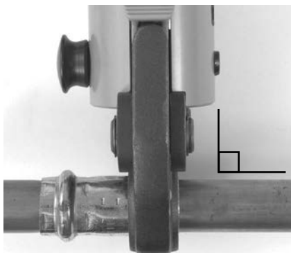
Obrázek 7 – Čelisti kolmo na armaturu
