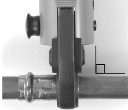
Εικόνα 7 – Κάθετη τοποθέτηση σιαγόνων στον σύνδεσμο
