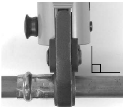
Slika 7 – Postavljane čeljusti pod pravim uglom u odnosu na priključak
