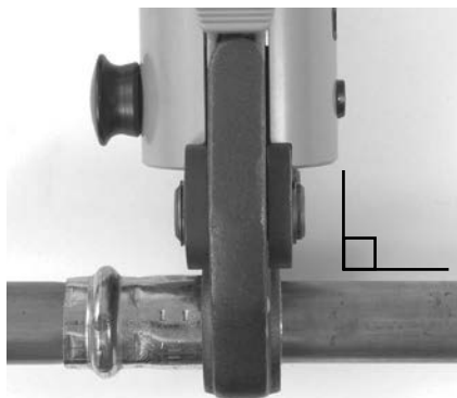
Figur 7 – Kæber, der er lige i forhold til fittingen
