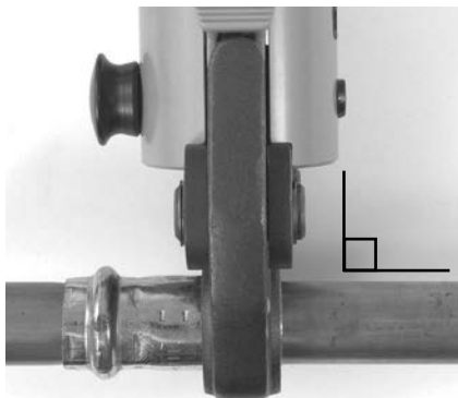
Slika 7 - Čeljusti pravokotno na nastavek
