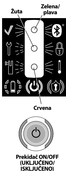
Slika 4 - Svjetla statusa alata
