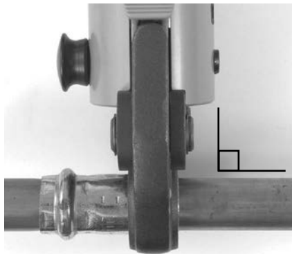
Figur 7 – Käftarna vinkelräta mot beslaget
