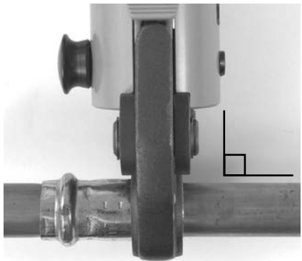
7. ábra – A pofák merőlegesen állnak a szerelvényre
