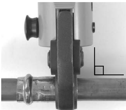
Рис. 7 – Пресс-клещи установлены перпендикулярно фитингу
