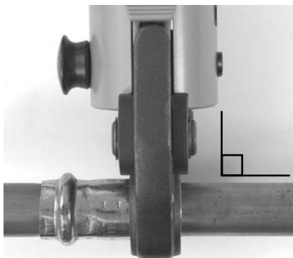
7-сурет – Фитингпен бір деңгейдегі қармауыштар
