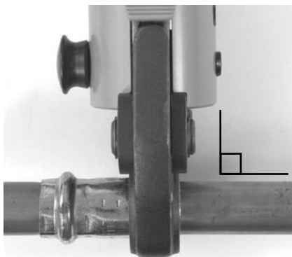
Rysunek 7 – Szczęki ustawione prostopadle do okucia
