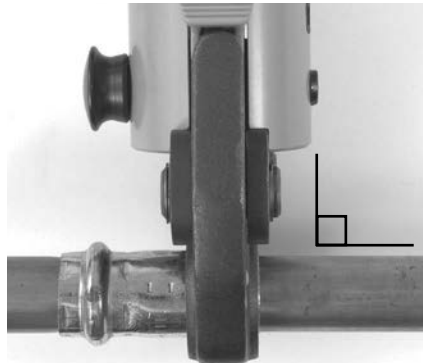
Kuva 7 – Leuat kohtisuorassa liittimeen
