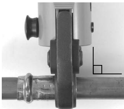
Figura 7 – Ganasce a squadra rispetto al raccordo
