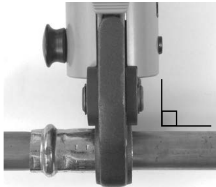
Slika 7 – Vilice pravilno postavljene na umetak
