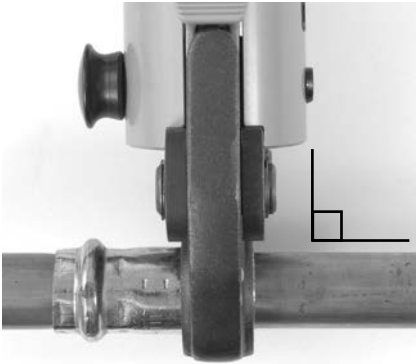
Figura 7 – La mordaza y el acoplamiento forman un ángulo recto
