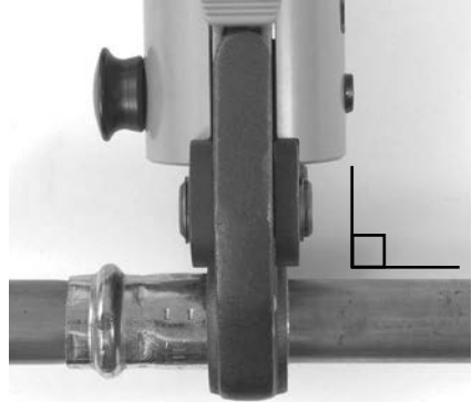
Şekil 7 – Çeneler Tespit Elemanına Dik
