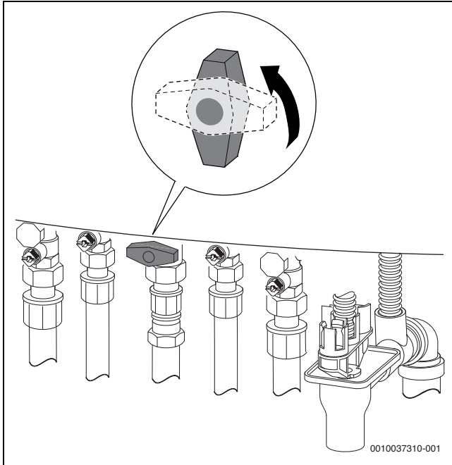
Fig. 6 Ouvrir le robinet gaz (vertical)
